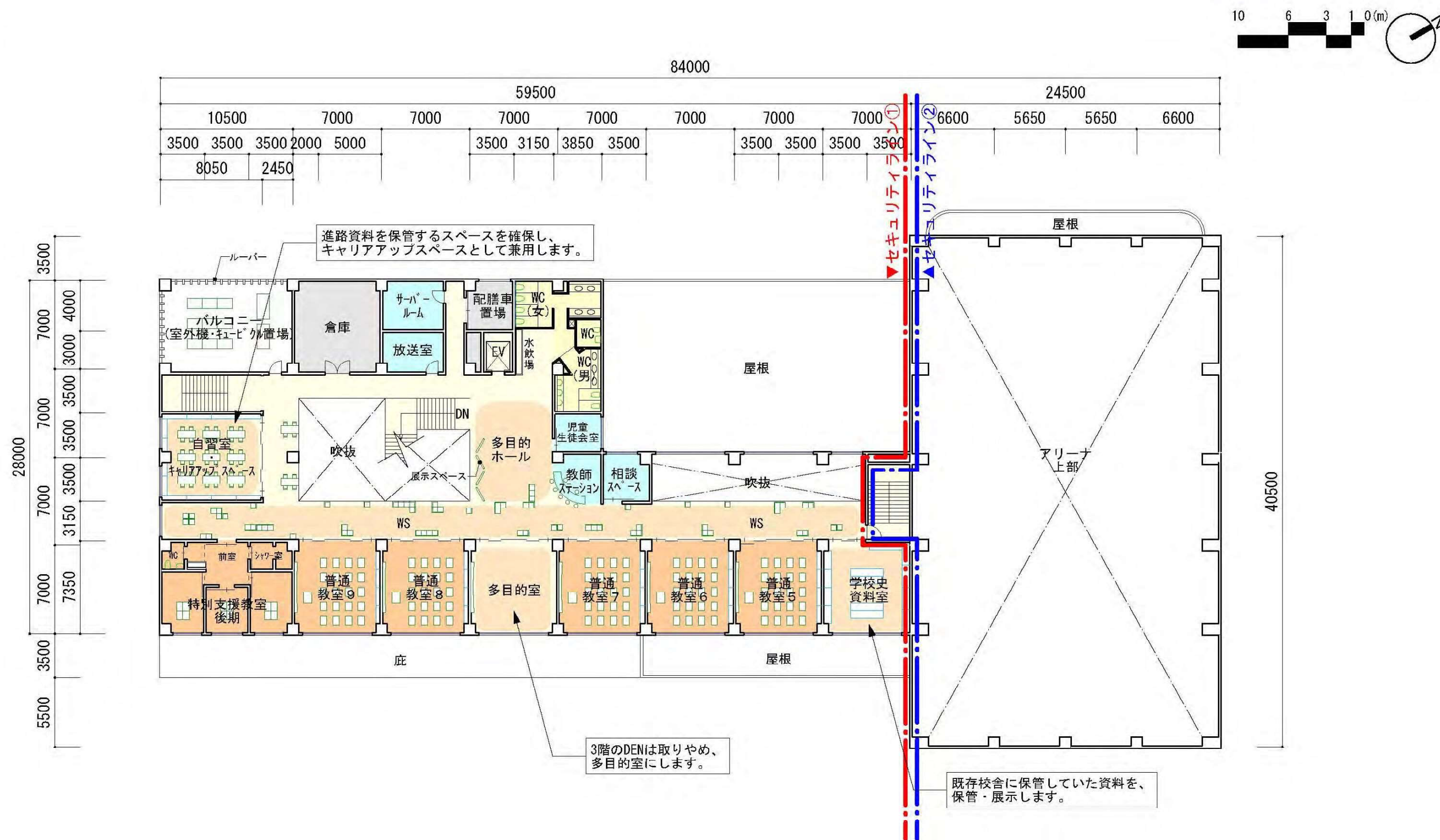
【3階平面図】
