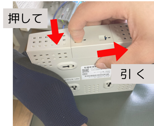
⑤上図のようにフタを垂直に 押しながら引く！
