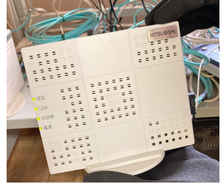
③ONU（白い箱状の機器）を確認
