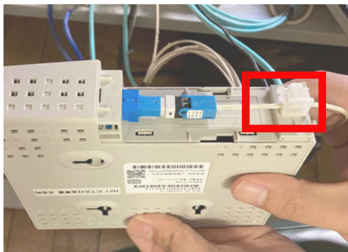
⑥白いつまみを外して、ケーブルを抜く 外したケーブルはまとめてくくっておくようにしてください
