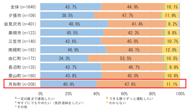
図 4-2 運転意向
